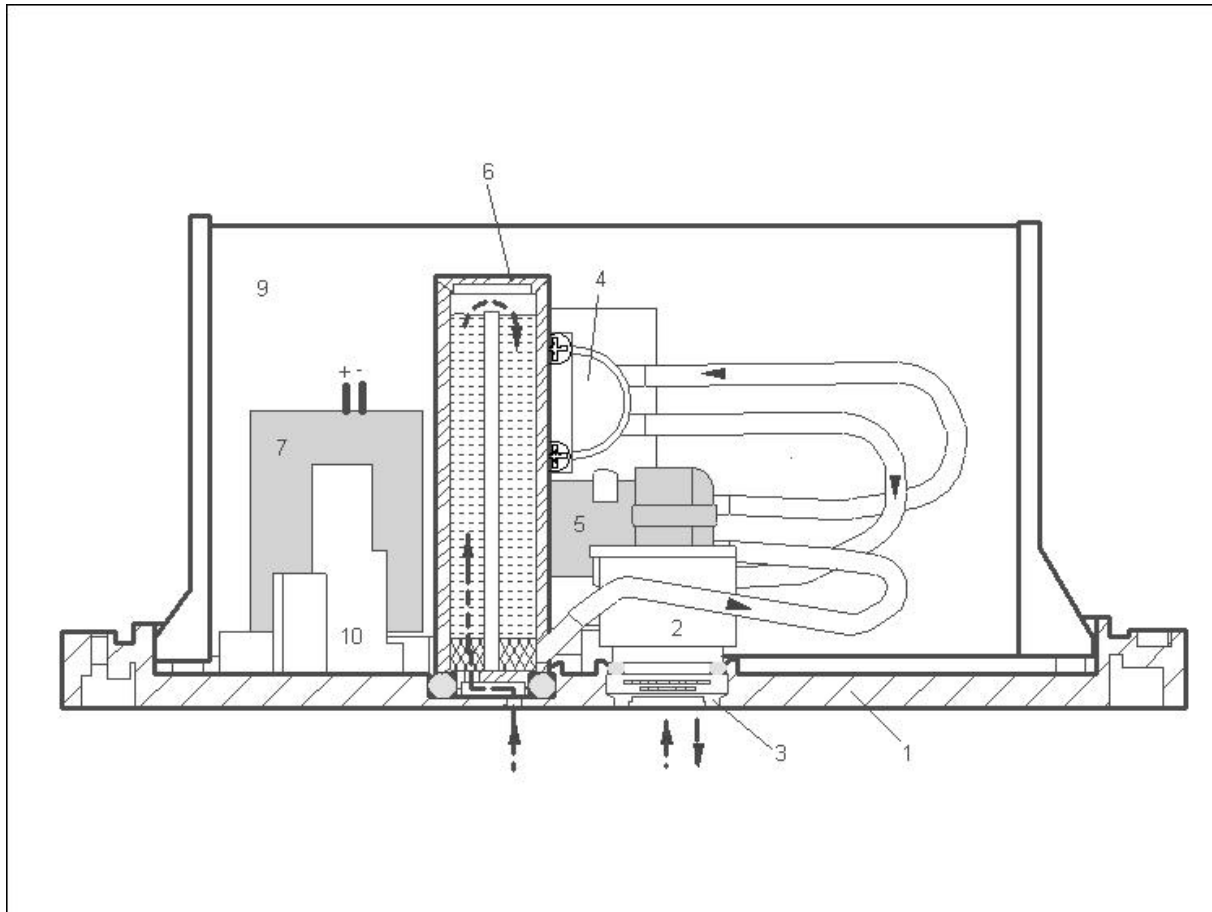
Abb. 2: Messkopf Statox 4120 für Cl 2 und ClO 2
