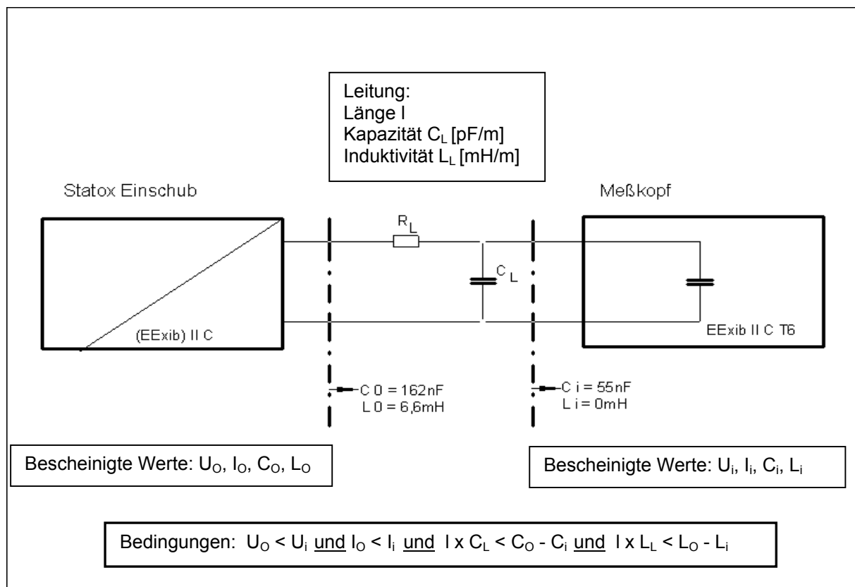
Abb.8: Zweidrahtleitung
