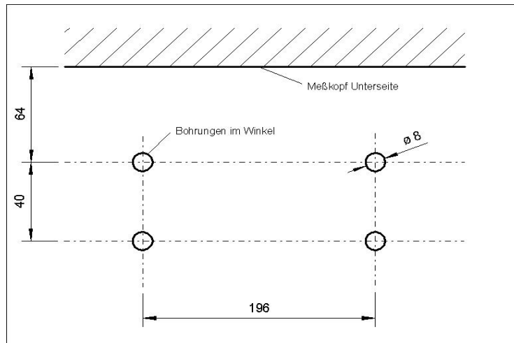
Abb.7: Bohrplan für die Montagewinkel des Statocx 4120 Messkopfes
