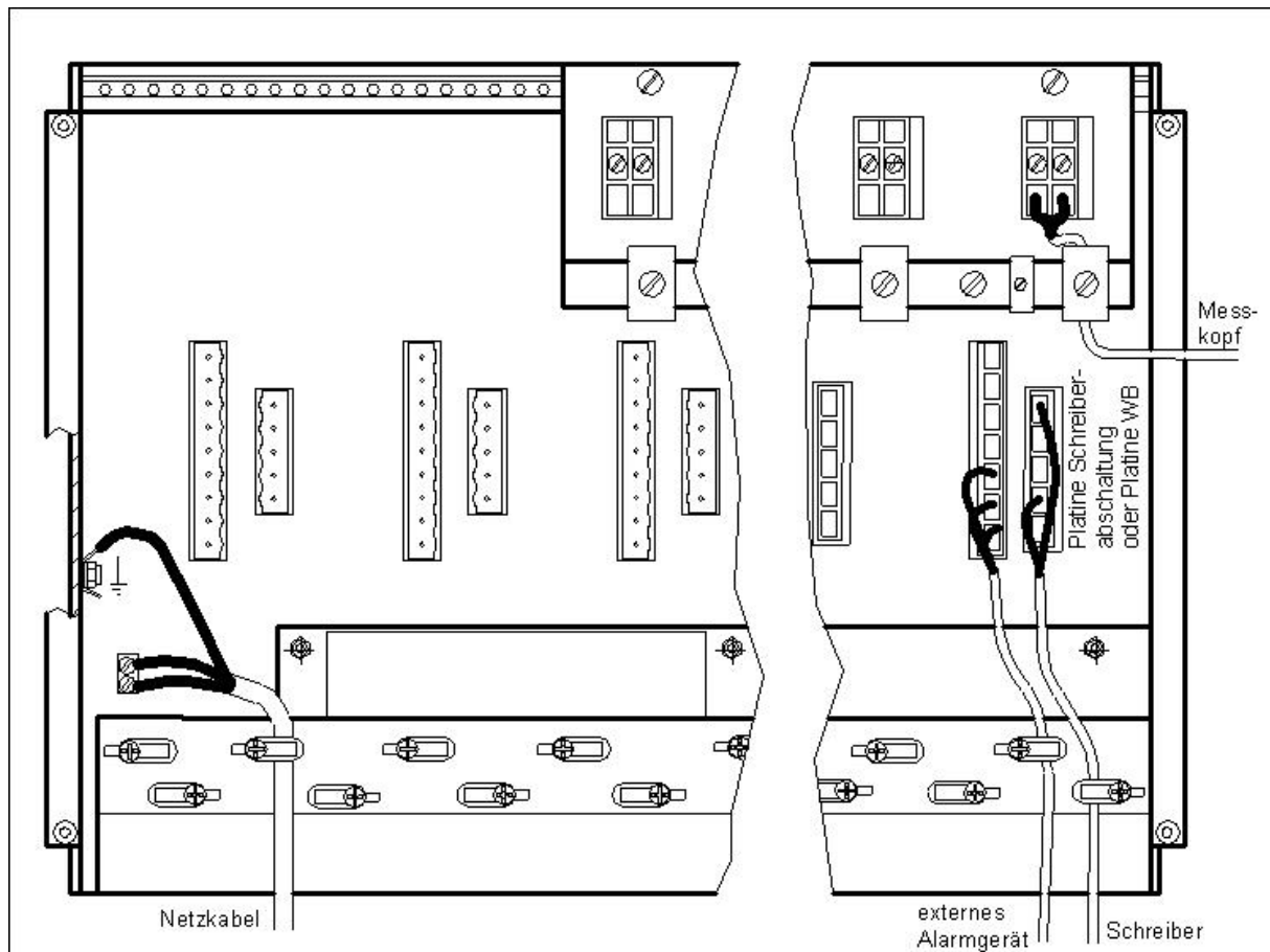
Abb.10: Rückseite Statox 4120 Rack
